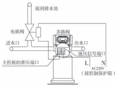
图3-11 泄压端口的接线图
