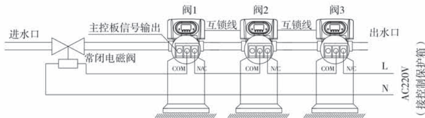
图3-5 多级串联时控制进口水电磁阀的接线图
