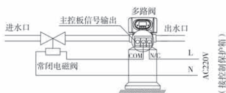
图3-3 控制进口电磁阀的接线图 图3-4 泄压端口的接线图
