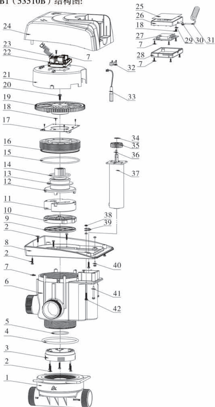
N75B1 (53510B) 结构图:
