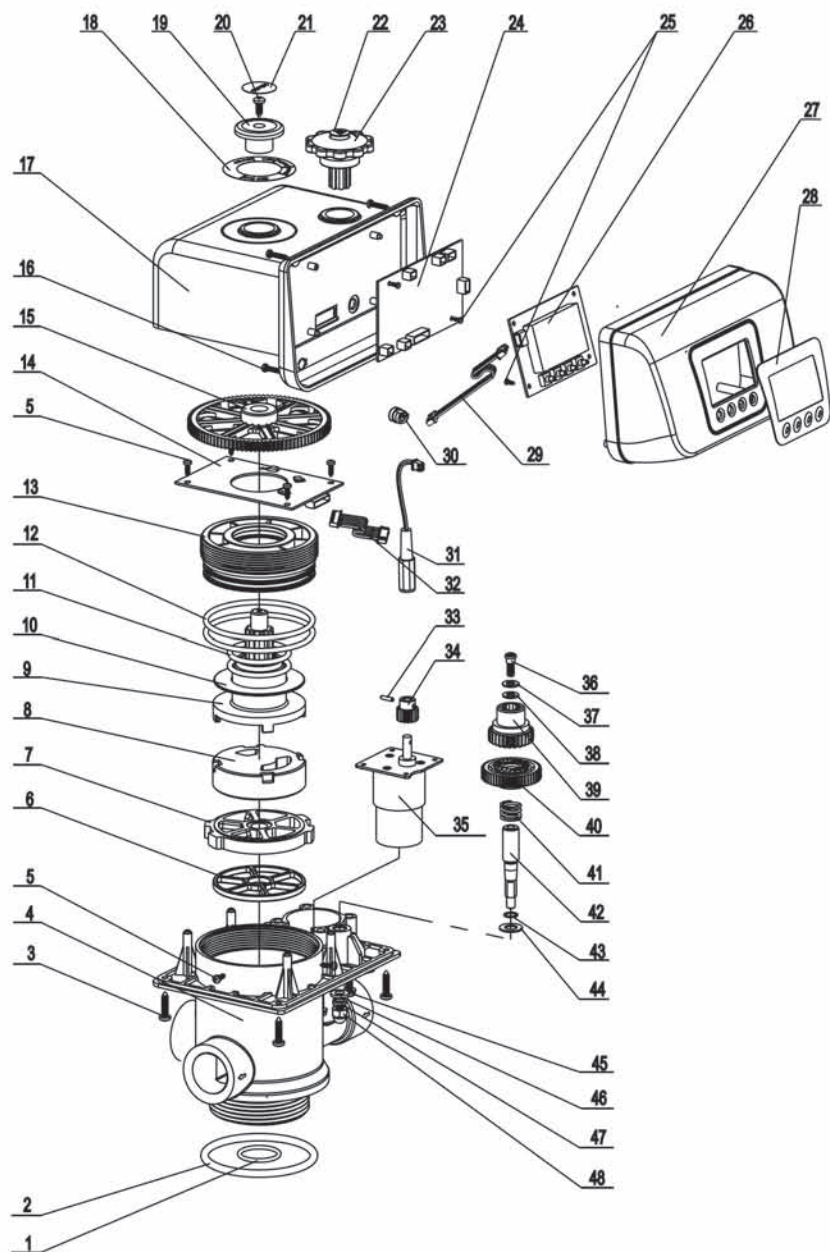
F67B1 (53504S) 结构图:
