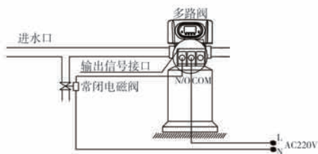
图3-3 控制进口电磁阀的接线图 图3-4 泄压端口的接线图
