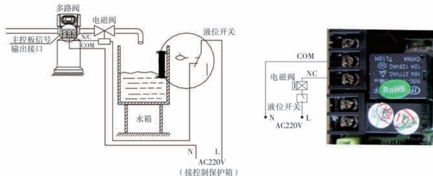
图3-1 控制出口电磁阀的接线图
