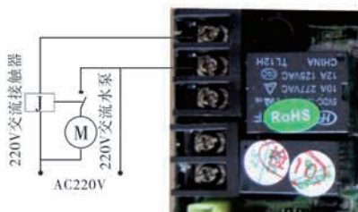
图3-8进口接增压泵的接线图
