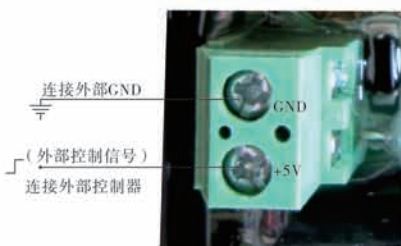
图3-11 远程控制端口的接线图
