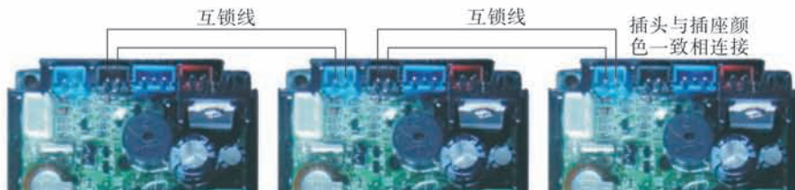
图3-9 互锁线接线图
