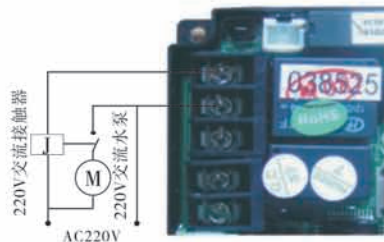
图3-8进口接增压泵的接线图
