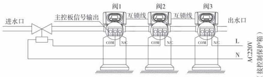
图3-4 多级串联时控制进口水电磁阀的接线图
