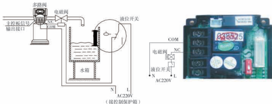
图3-1 控制出口电磁阀的接线图
