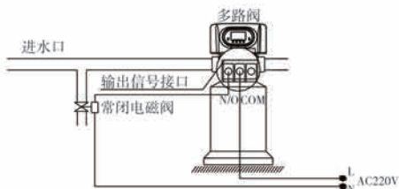
图3-3 泄压端口的接线图
