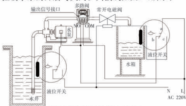
图3-5 通过水箱液位控制进水泵的接线图
