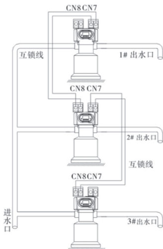
图3-12 同时供水，分别再生
