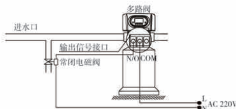
图3-3 泄压端口的接线图
