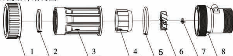
5447003流量计零部件名称及编码:
