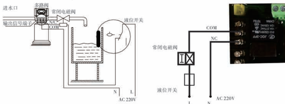
图3-1 控制出口电磁阀的接线图
